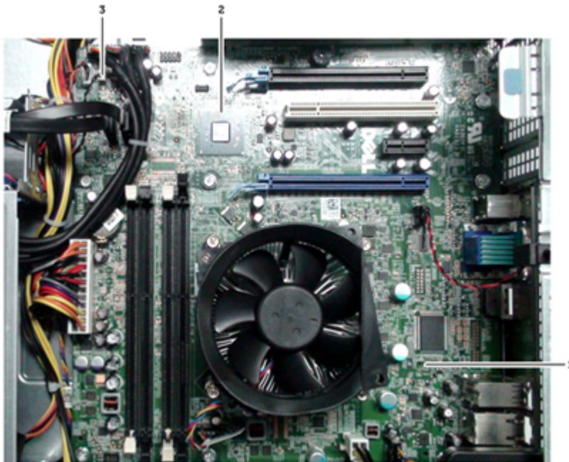
2. ábra. Alaplap eltávolított hőérzékelővel és hűtőbordával
