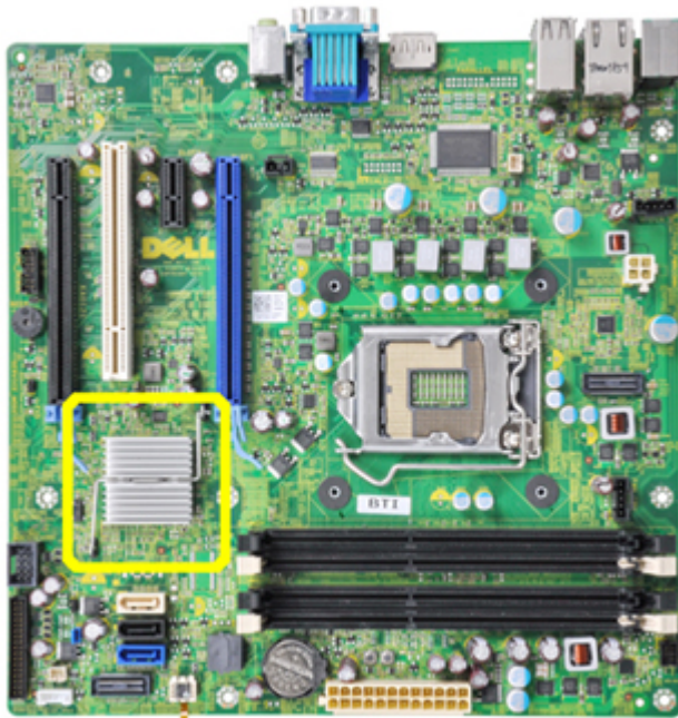
1. ábra. Korábbi verziójú alaplap hűtőbordával
